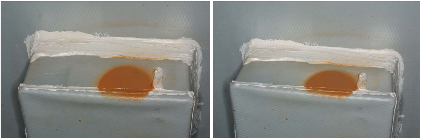
Figur 3. Prøveemne med firkantet gennemføringsselement i aluzink før (til venstre) og efter (til højre) påvirkning i By og Bygs klimasimulator.
